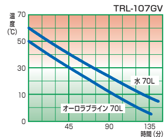
冷却能力表 TRL-107GV
