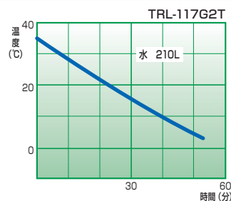
冷却能力表 TRL-117G2T
