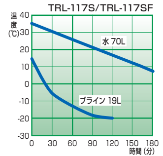
冷却能力表 TRL-117S/TRL-117SF
