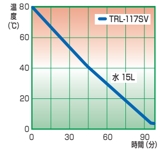
冷却能力表 TRL-117SV/TRL-117SFV
