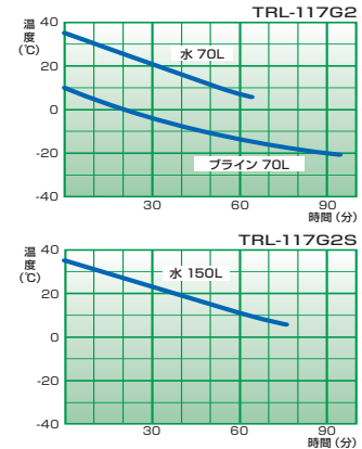
冷却能力表 TRL-117G2
