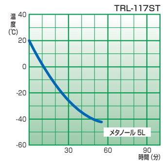
冷却能力表 TRL-117ST
