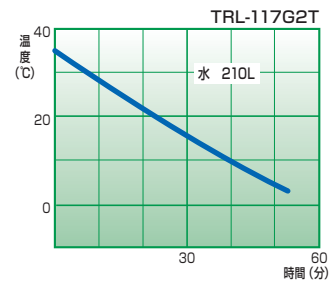
冷却能力表 TRL-117G2T
