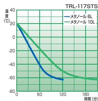
冷却能力表 TRL-117STS
