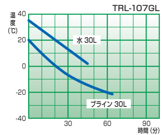
冷却能力表 TRL-107GL
