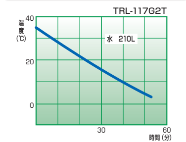
冷却能力表 TRL-117G2T
